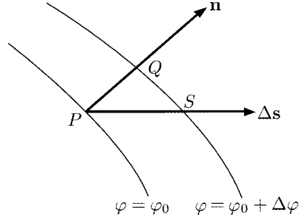
Σχήμα 1.3: Τμήματα δύο ισοδυναμικών επιφανειών της συνάρτησης \varphi(x, y, z) . Το |\text{grad } \varphi| στο σημείο P είναι ίσο με το όριο του \Delta\varphi/\overline{PQ} , καθώς το \overline{PQ} \rightarrow 0 , και το d\varphi/ds είναι το αντίστοιχο όριο του \Delta\varphi/\overline{PS} .
