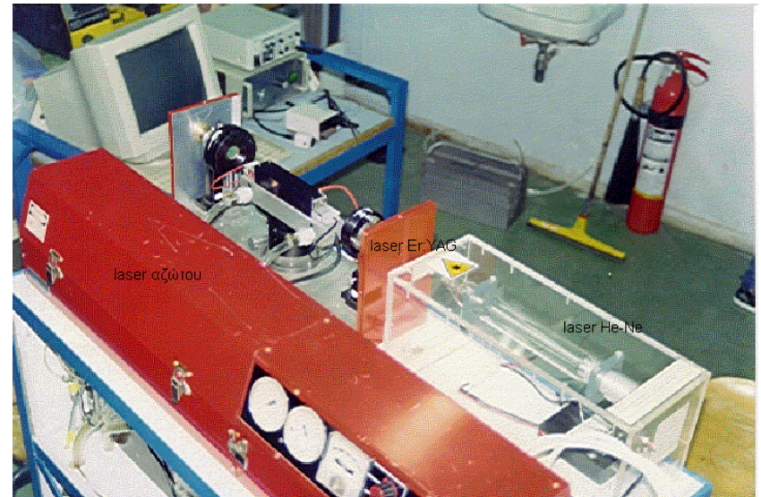
Διακρίνεται η κεφαλή του επεμβατικού laser Er:YAG, το laser-οδηγός (He-Ne) και το laser αζώτου για τη φασματοσκοπία επαγόμενου φθορισμού.
