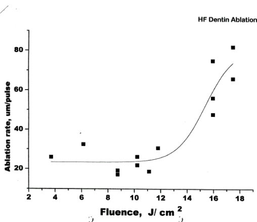
Ρυθμός αποδόμησης της οδοντίνης ως συνάρτηση της πυκνότητας ενέργειας laser στα 2,94 \mu\text{m} .
