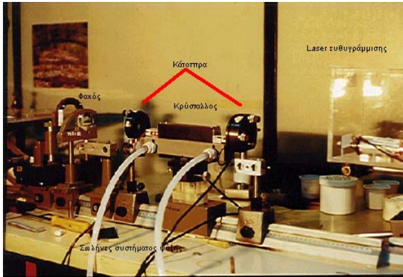
Εργαστηριακό πρωτότυπο Er:YAG laser – κεφαλή.
