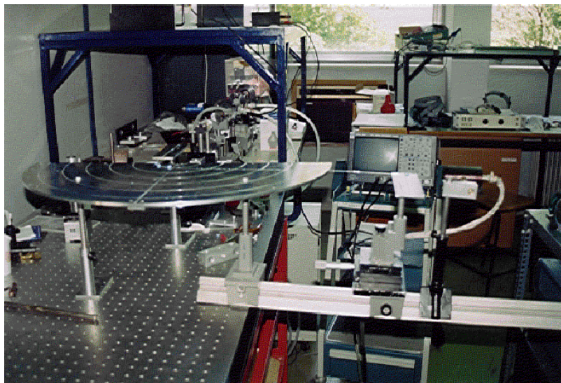
Μετρήσεις διέλευσης της δέσμης του laser Er:YAG μέσα από οπτική ίνα.
