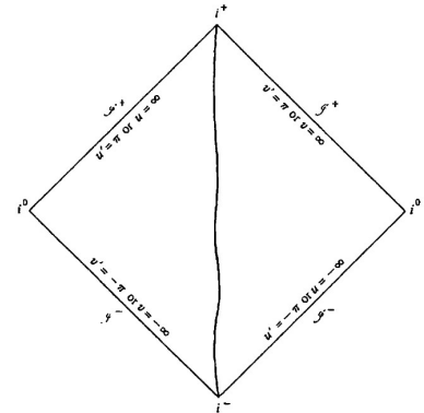
Σχήμα 4.4: Διάγραμμα Penrose για Minkowski
