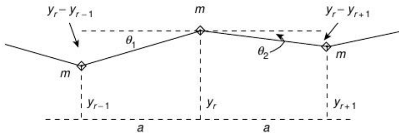
Σχήμα 2.1: Μέθοδος Lagrange προσομοίωσης συνεχούς χορδής.
