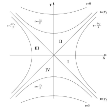
Σχήμα 4.1: Κώνος Φωτός σε συντεταγμένες Rindler
